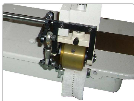
Particolare del puller della SIMAC 1721 - P Detail of the puller of SIMAC 1721 - P
